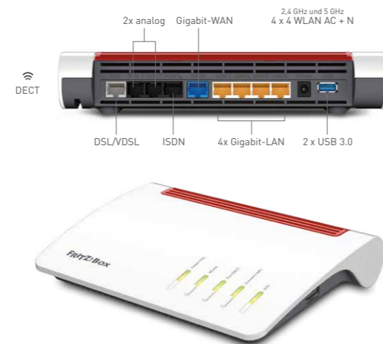
Abb. 4 Router und Anschlüsse
